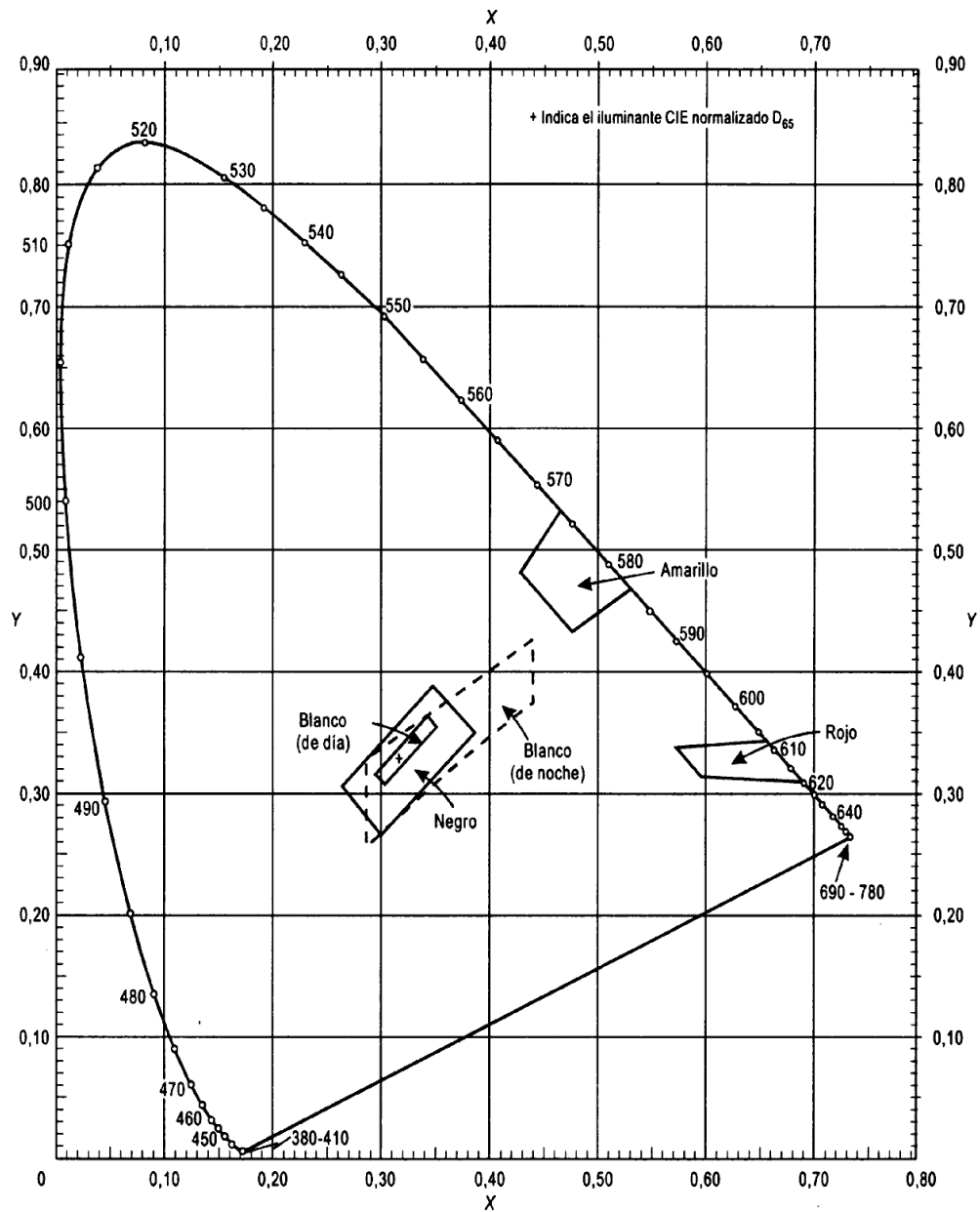
Figura A1 - 4. Colores de los letreros y paneles transluminados ( Iluminación interna )
